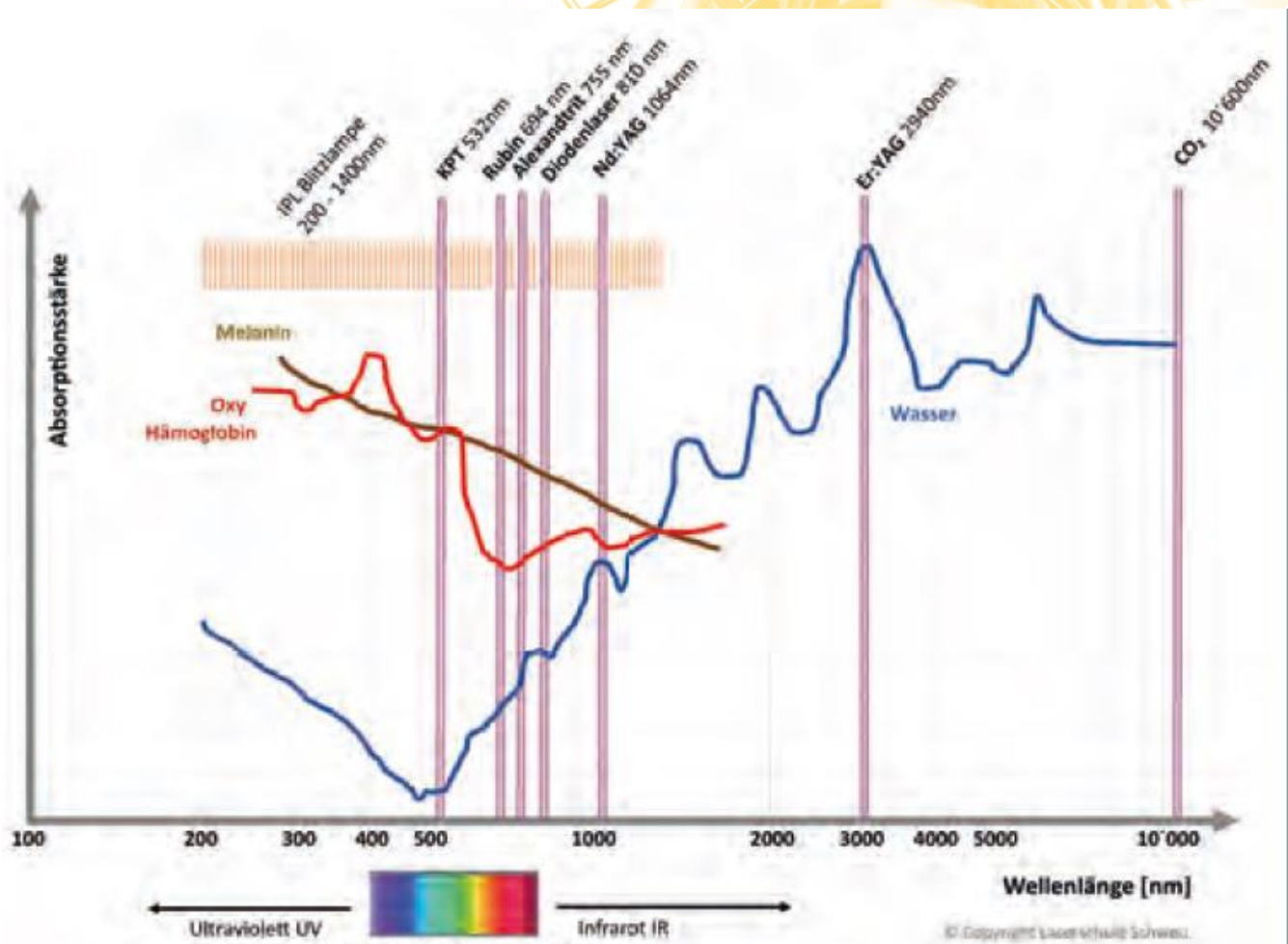
Übersicht, welcher Stoff (Blut, Wasser, Melanin) von welcher Wellenlänge wie stark absorbiert wird. Auszug aus unserem Bericht für die SGMK, Ausgabe 4/2018 und freundlicher Genehmigung der Laserschule Schweiz www.laserschule.ch
